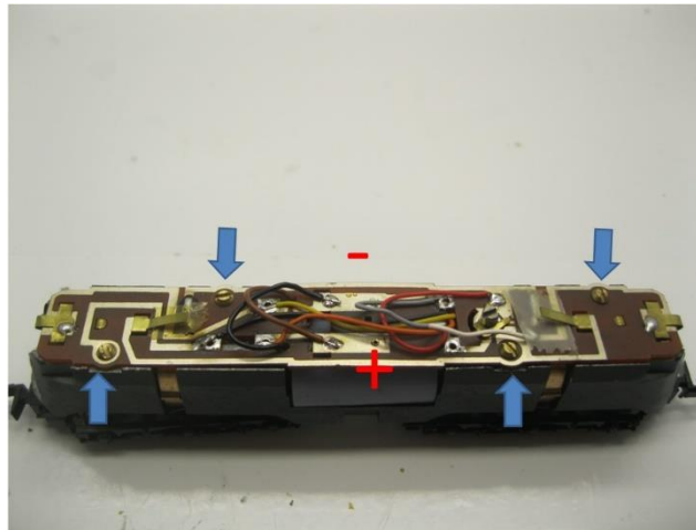
Platzieren Sie die Platine und löten Sie die Drähte Mount the PCB and solder the wires Plaats de printplaat en soldeer de draden
