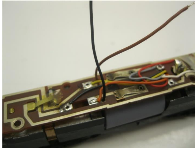
Bohren Sie 2 Löcher für die Drähte Drill 2 holes for the wires Boor 2 gaten voor de draden
