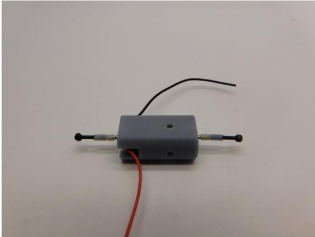
Kardankupplungs platzieren Mount the cardan couplers Plaats de cardan koppelingen
