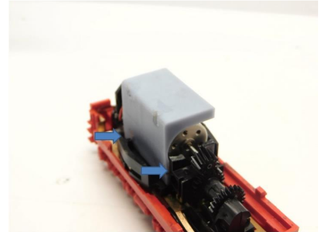
Damit sich der Motor nicht verschiebt, wird er mit 2 Tropfen Kleber gesichert So that the motor does not shift, it is secured with 2 drops of glue Verlijm de motor met 2 druppels lijm zodat deze niet verschuift
